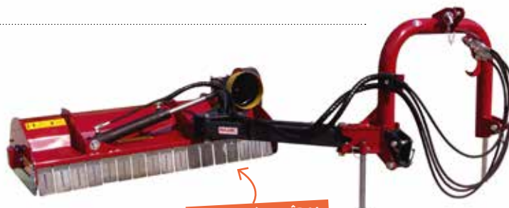
ROTOR HÉLICOÏDAL
